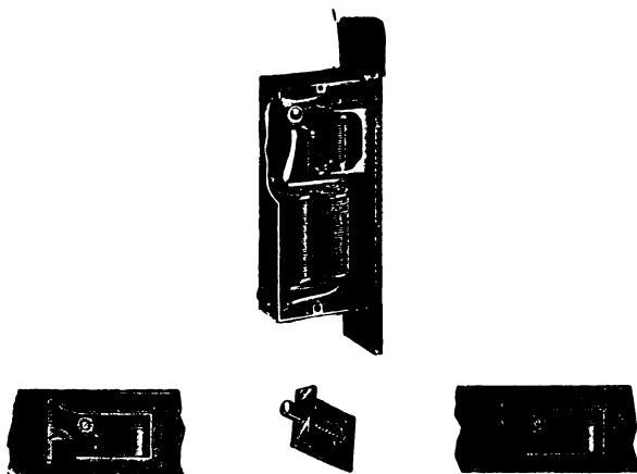
FIG. 62.—ELECTRIC DOOR-OPENER.
