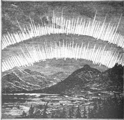
FIG. 91.—AURORA BOREALIS.
